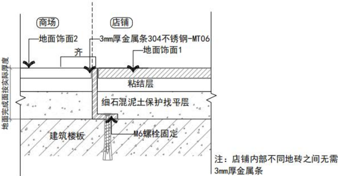
01 | 商场与店铺地面齐平金属过渡详图 SHT NO. SCALE: 1:2
