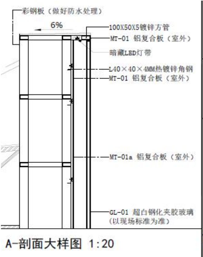
入口门头节点图
