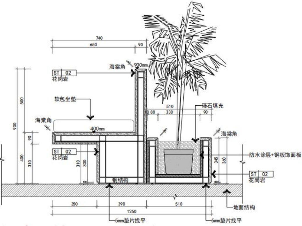
长凳+花槽M-1-10a&M-3-20剖面图
