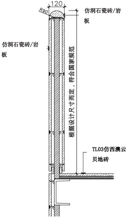
栏杆详图
