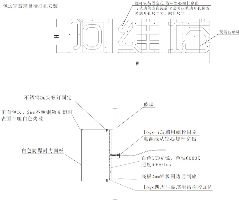
包边字 英文发光LOGO 玻璃幕墙钢结构安装
