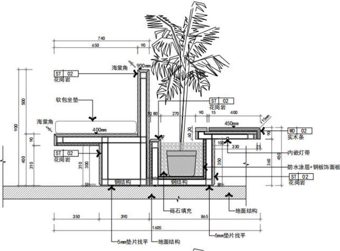
长凳+花槽M-1-10a&M-3-20剖面图
