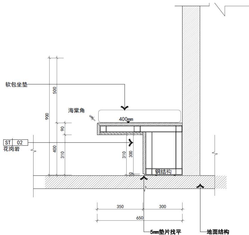
长凳+花槽M-3-20b剖面图
