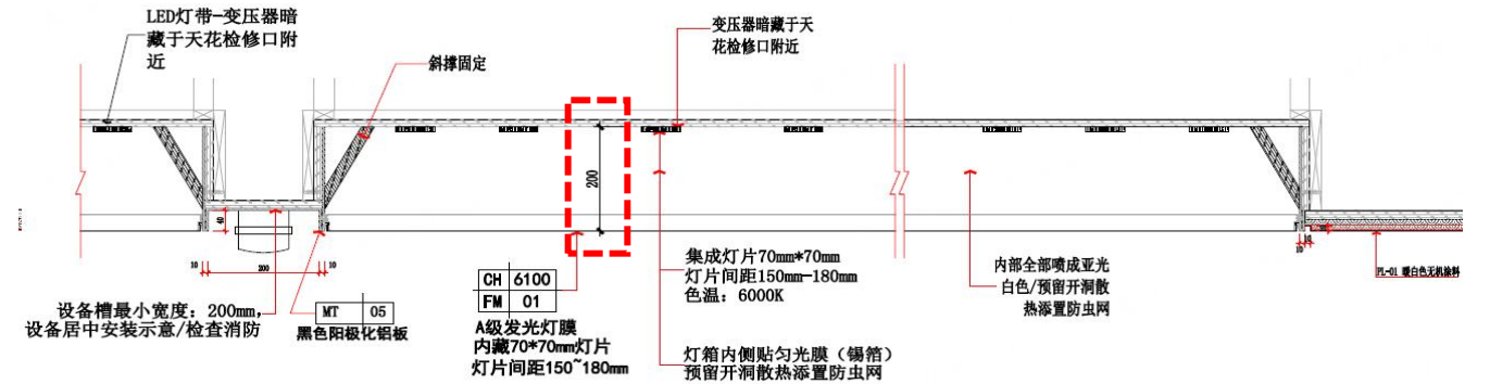
04 展厅吊顶灯膜剖面图
