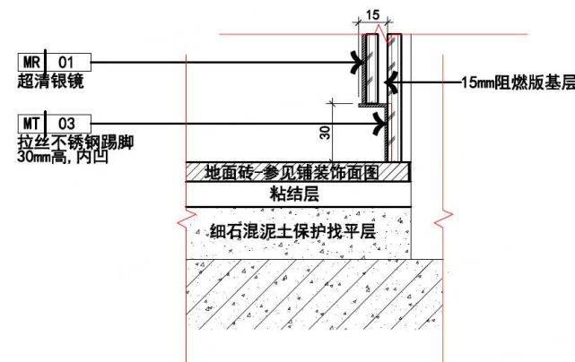
02 银镜墙剖面图
