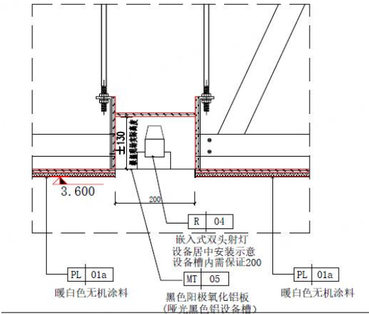
A D-02 天花板节点 大样图 SCALE 1:8
