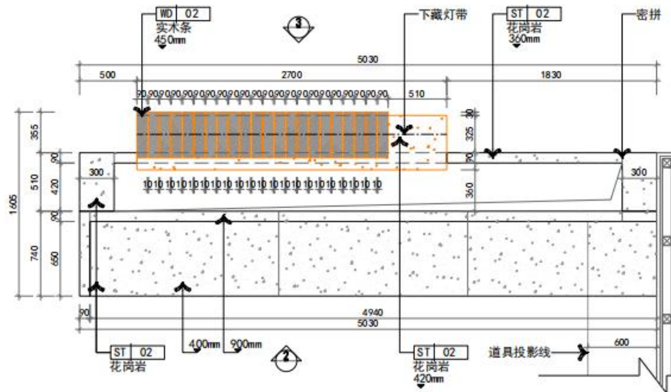
01 | 长凳+花槽M-1-10a&M-3-20平面图
