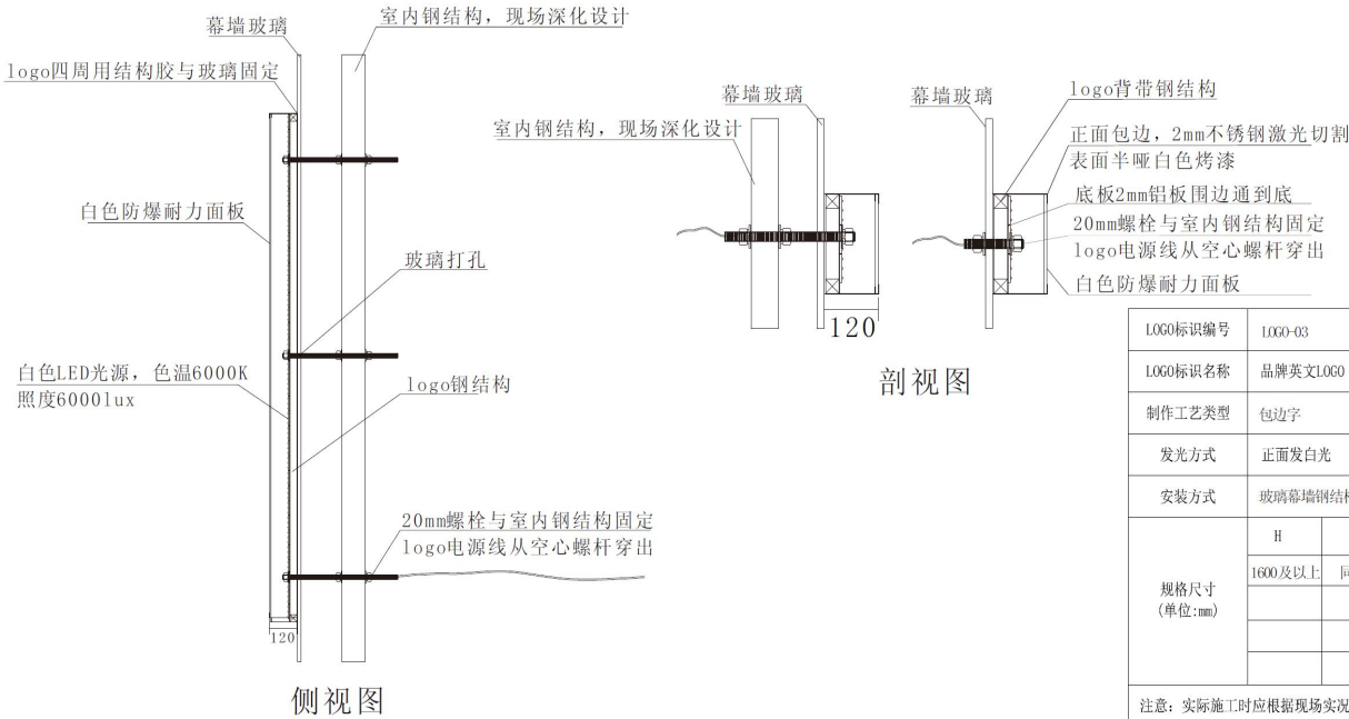
标识安装节点图
