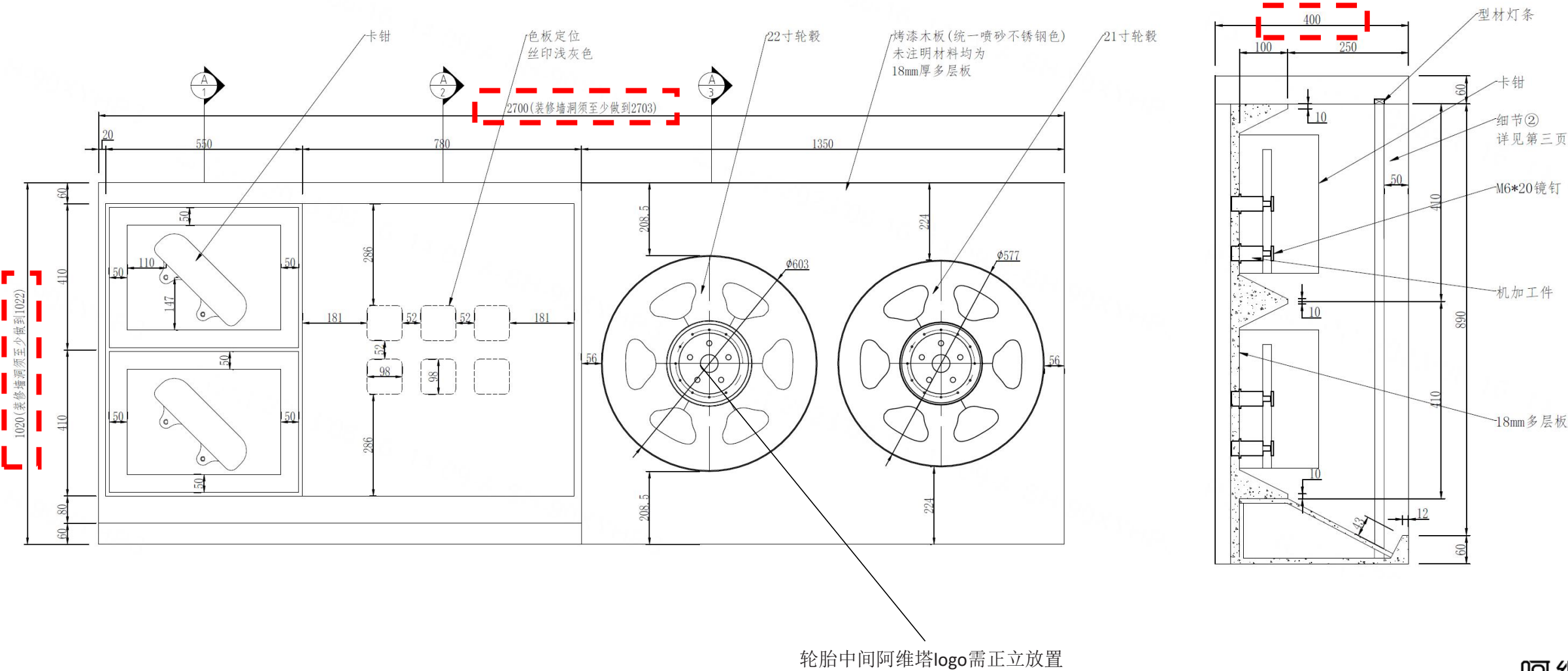
4.2.2 街道CMF柜节点图
