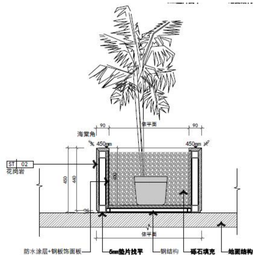
04 | 长凳+花槽M-3-20剖面图
