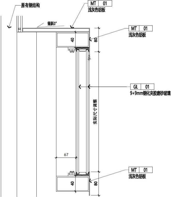
02 外立面玻璃造型节点做法 1:5
