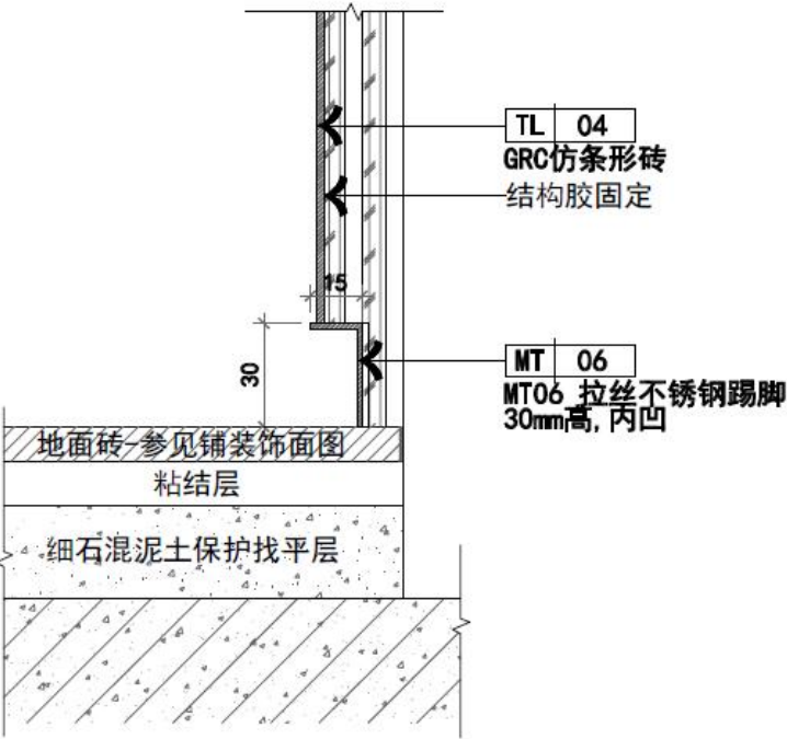
03 | GRC室内墙剖面图 SHT NO. SCALE: 1:2
