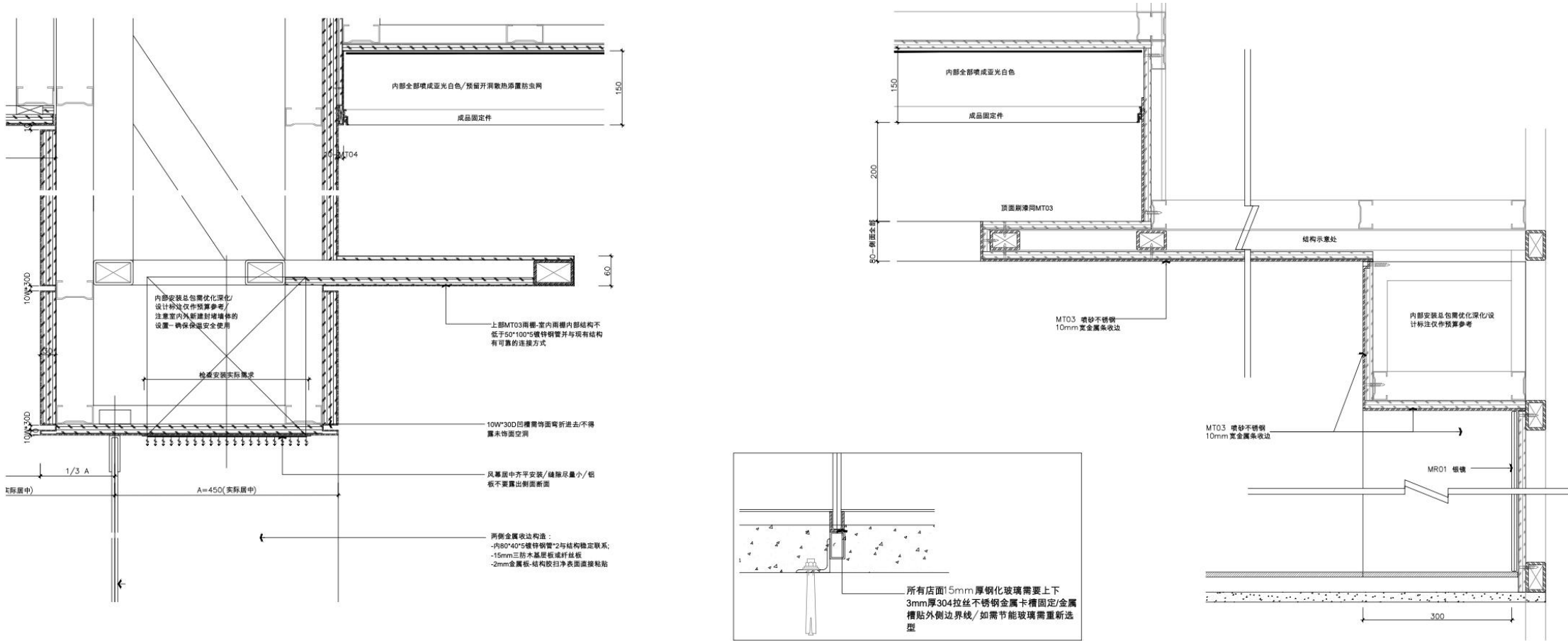
玻璃及室内不锈钢雨棚节点
